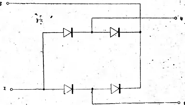
Схема электрическая принципиальная микросхемы 2Д906А
