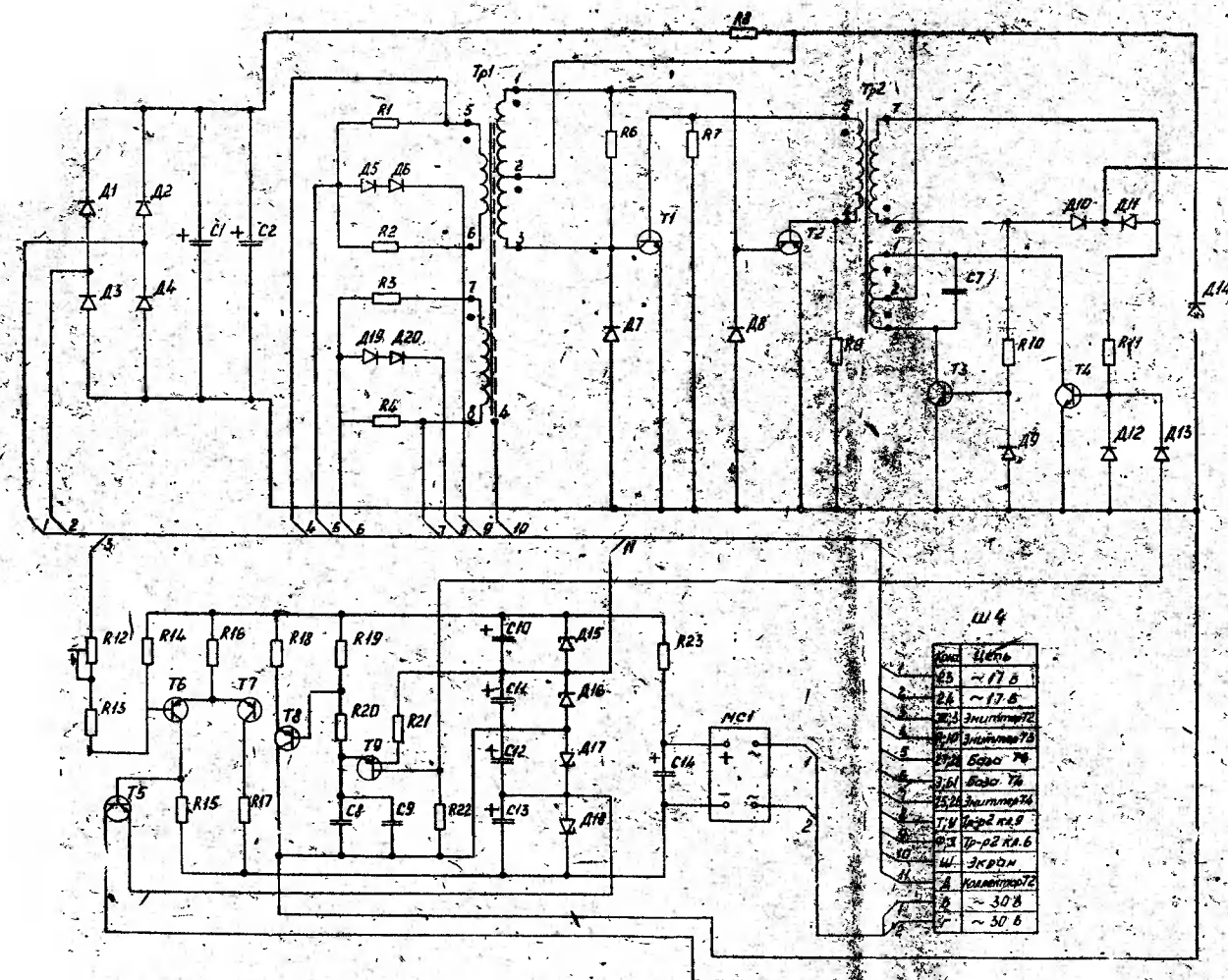
Схема электрическая принципиальная платы 3.660.012-Э3
