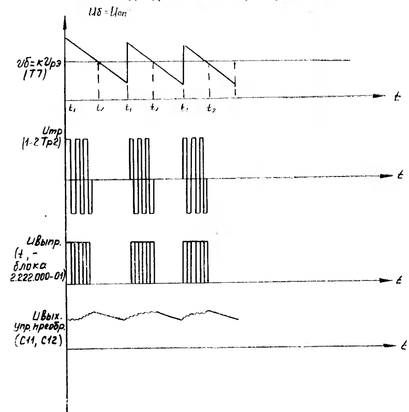
Рис. 12. Эпюры напряжения на элементах управляемого преобразователя
