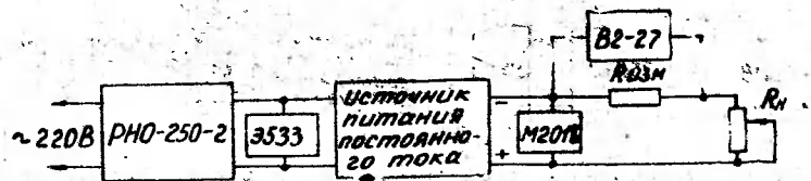
Рис. 8. Структурная схема измерения частной неустойчивости выходного тока от изменения напряжения питающей сети в режиме стабилизации тока
