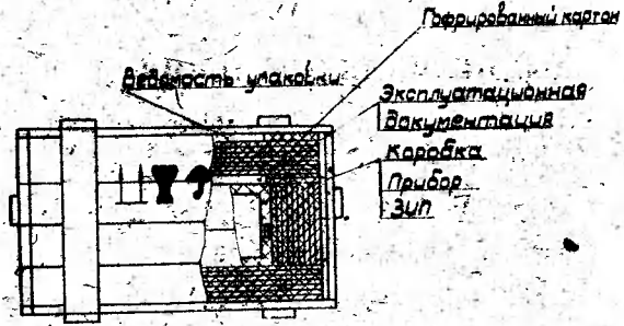
Рис. 16. Упаковка источников питания при транспортировании
