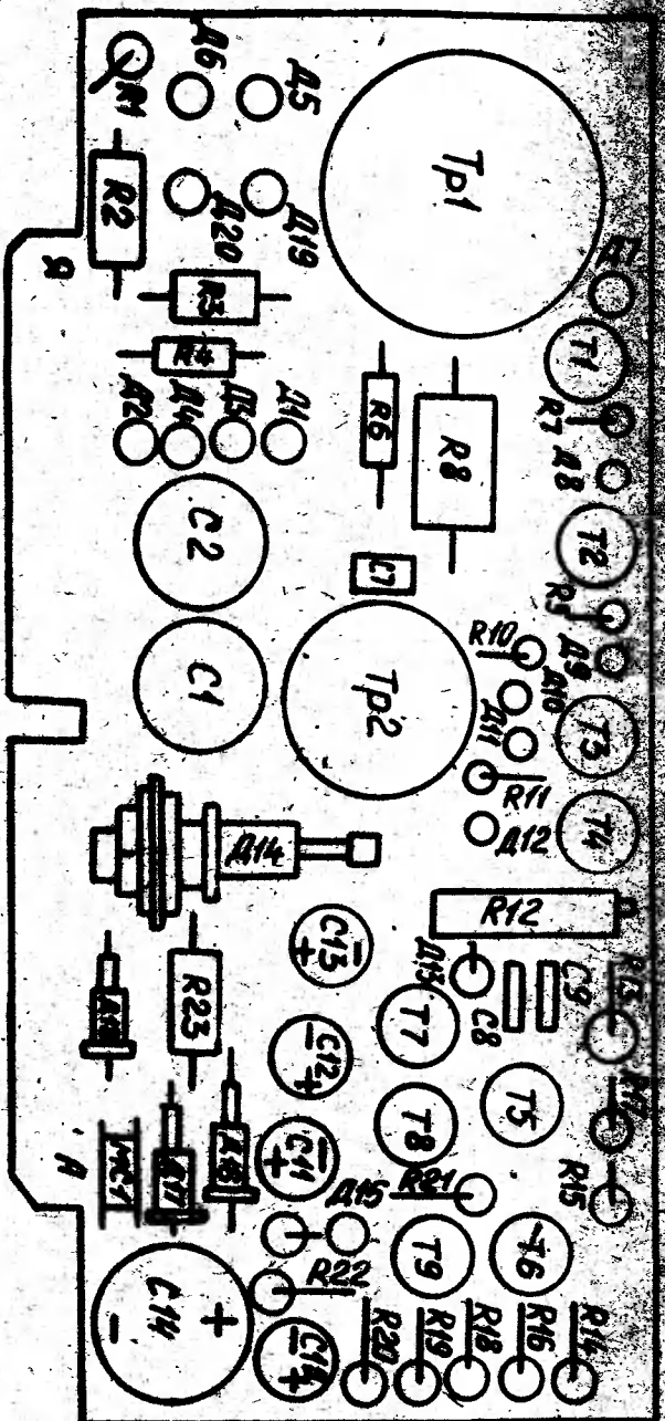
Размещение элементов на плате 3.660.012
